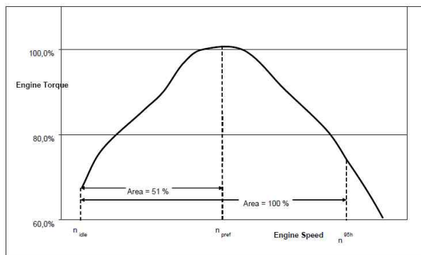
그림 4. N_{pref} 회전수의 정의
