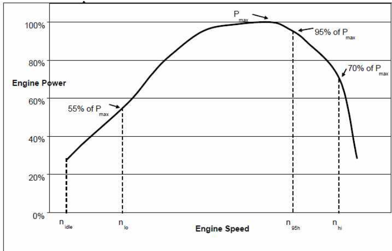
그림 4. N_{pref} 회전수의 정의
